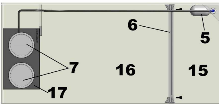
Schéma 1a : Cuve de filtration Armatus Lagoon 400
