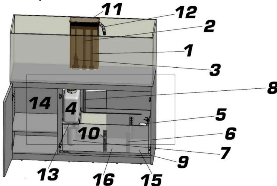
Abb. 1: Überlauf und Unterschrankfilter
