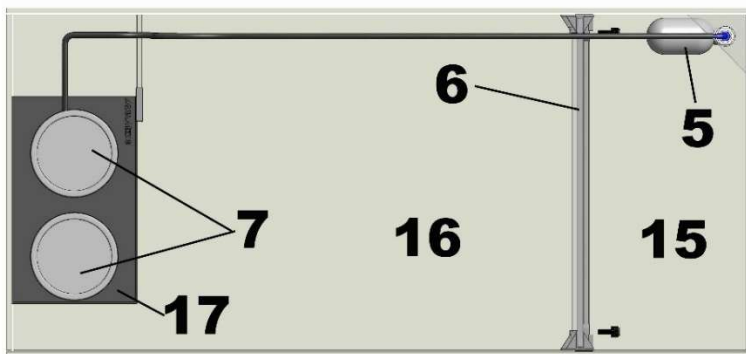
Rys. 1a: Zbiornik filtracyjny Armatus Lagoon 400
