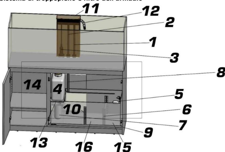
Fig. 1: Sistema di troppopieno e filtro dell'armadio
