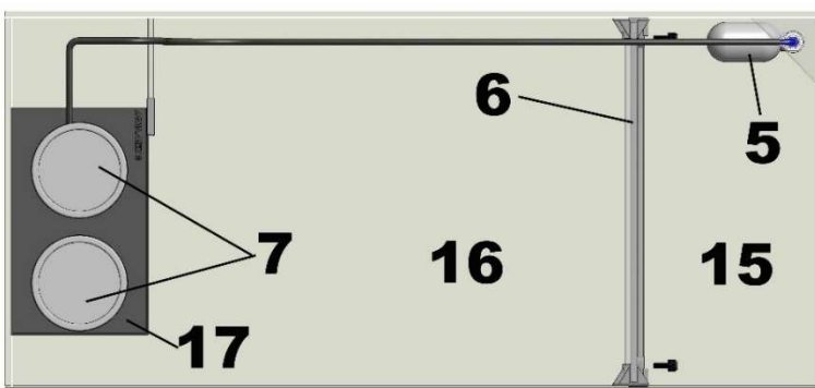
Fig. 1a: Sumidero de filtro Armatus Lagoon 400
