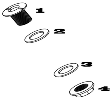
Fig. 3: Collegamento a vite passante o a serbatoio (la lastra di vetro si trova tra l'anello scorrevole 3 e l'anello di gomma 2).
