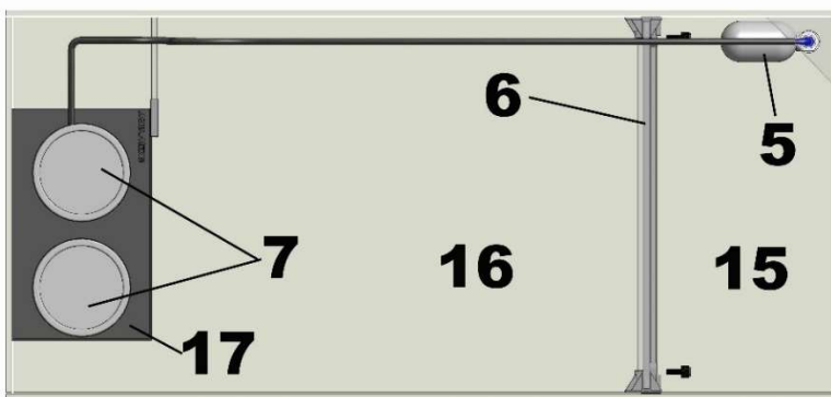
Fig. 1a: Bacino filtrante Armatus Lagoon 400
