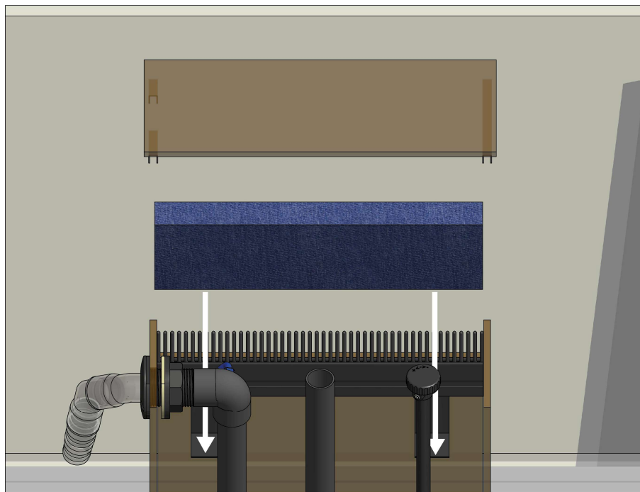
Fig. 4: Traboccare con la spugna e coprire
