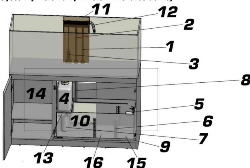
Rys. 1: System przelewowy i filtrem w szafce dolnej
