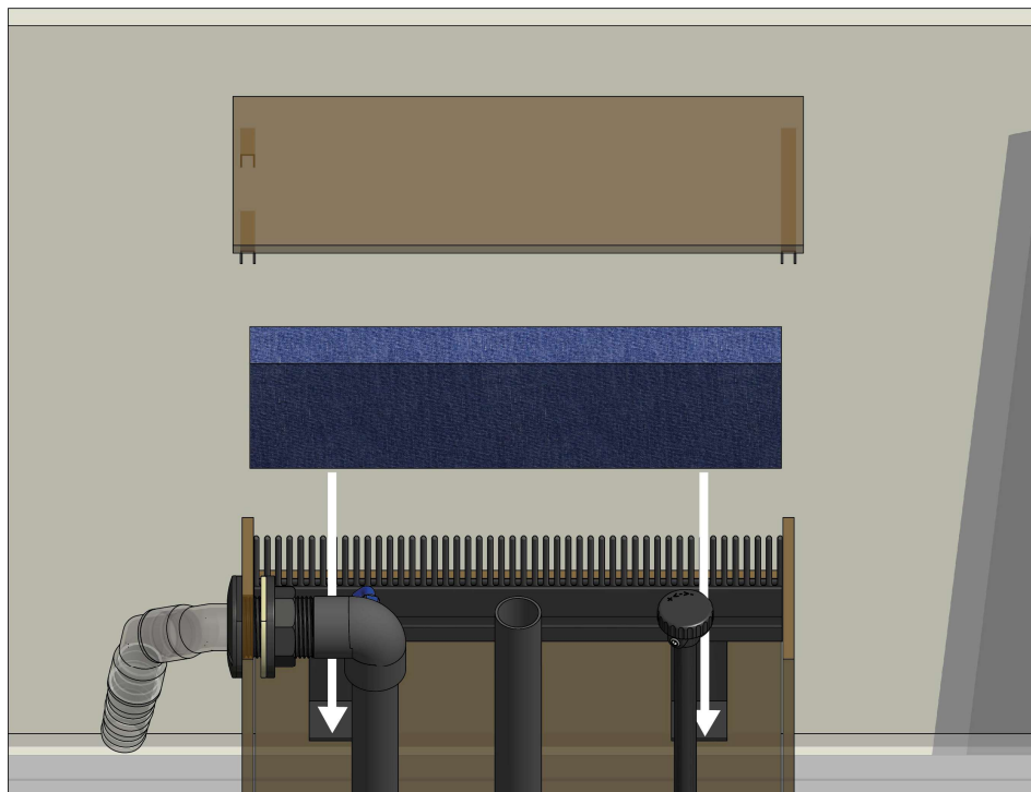
Рис. 4: Перелив с губкой и крышкой
