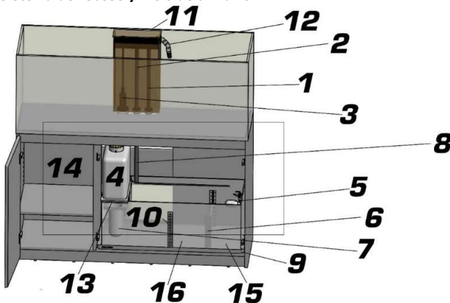
Fig. 1: Filtro de rebose y de armario
