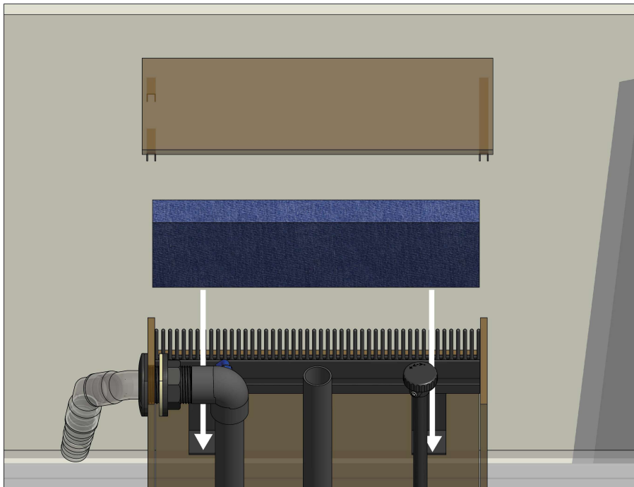
Abb. 4: Überlauf mit Schwamm und Abdeckung
