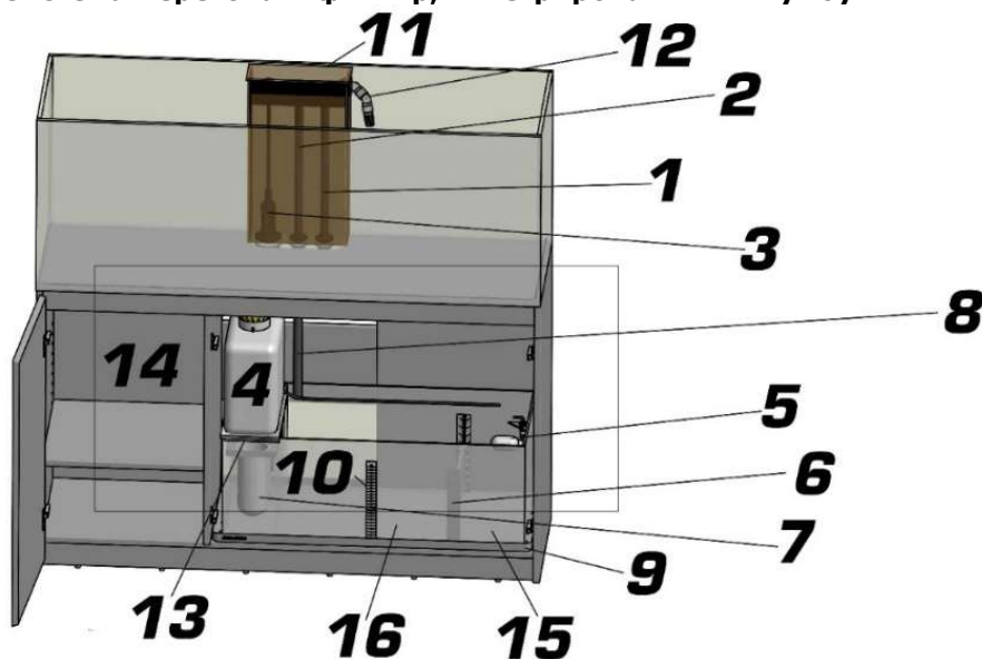
Рис. 1: Переток и фильтр, интегрированный в тумбу
