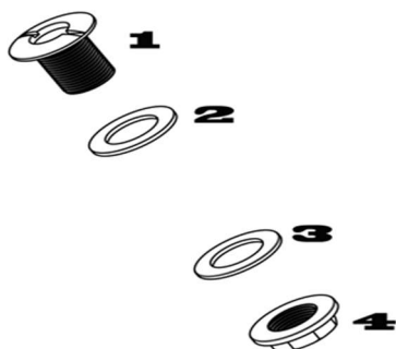
Rys. 3: Przepust szczelny (przelot przez szkło) (szyba znajduje się między pierścieniem ślizgowym 3 i pierścieniem gumowym 2)
