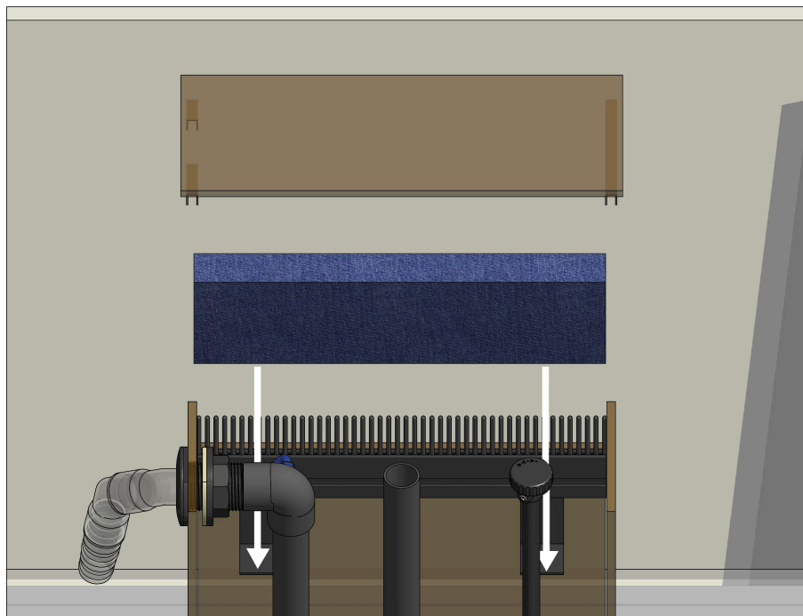
Rys. 4: Przelew z gąbką oraz przykrywka
